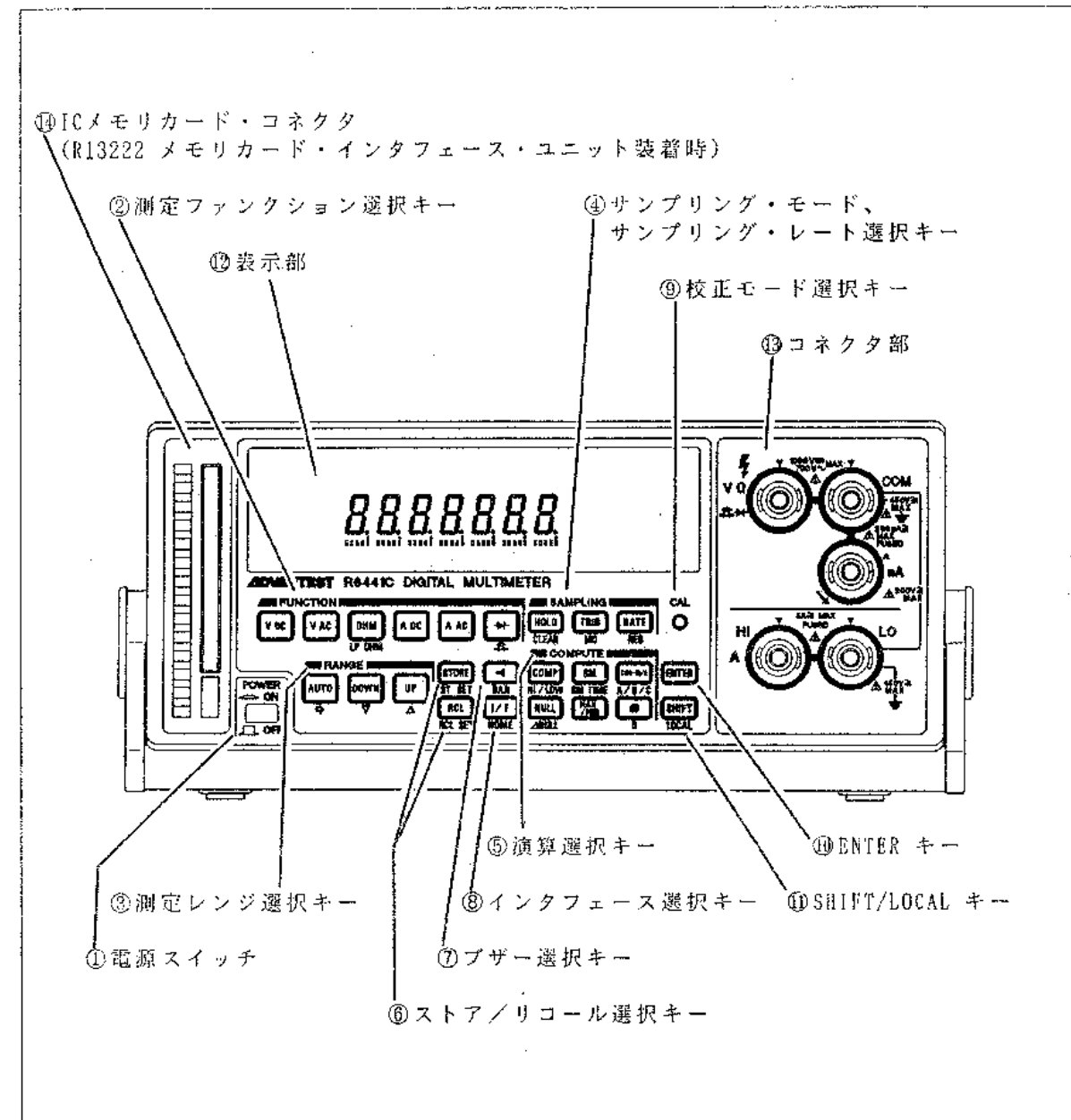
図 3 - 3 R6441C 正面パネルの説明
