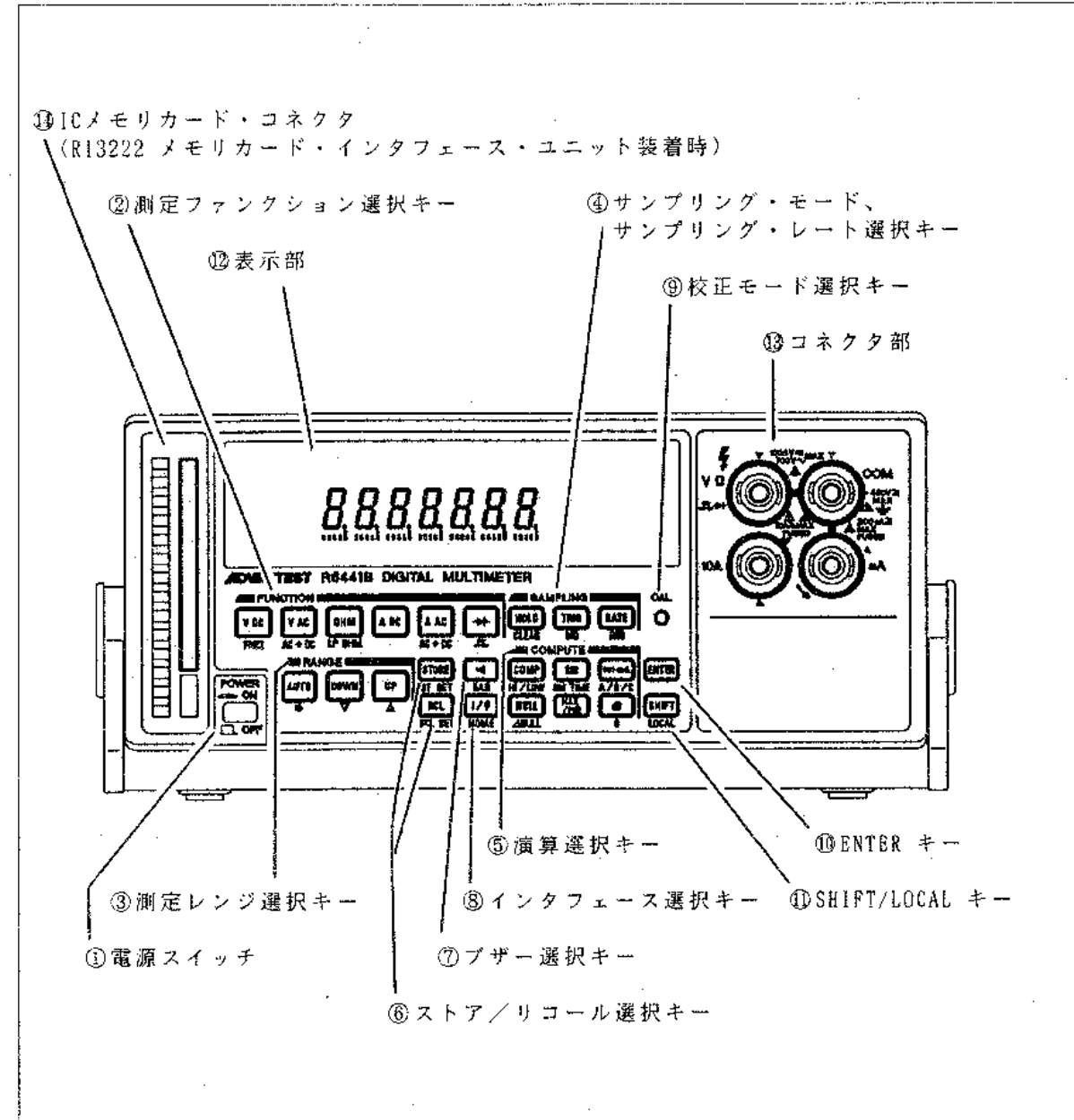
図 3 - 2 R6441B 正面パネルの説明
