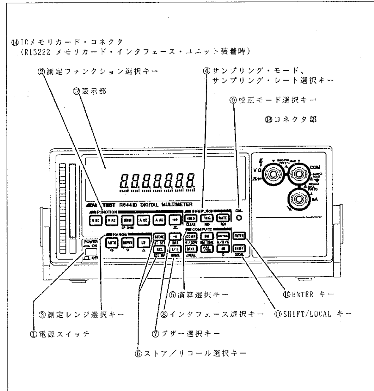
図 3 - 4 R6441D 正面パネルの説明
