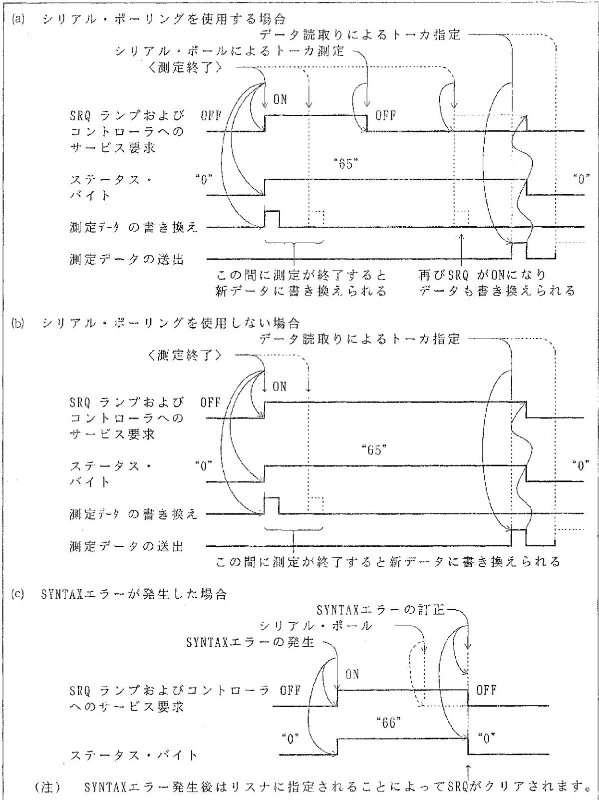
図 7 - 4 サービス要求時の動作タイミング
