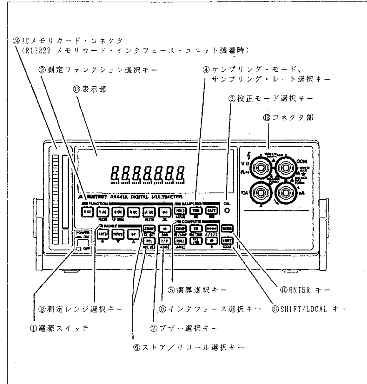
図 3 - 1 R6441A 正面パネルの説明
