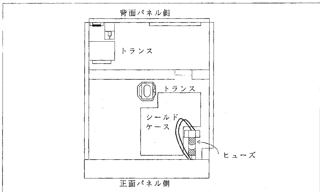
図 2 - 5 A 入 力 端 子 保 護 用 ヒ ュ ー ズ
