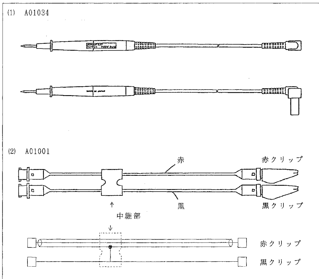
図 2 - 6 入力ケーブルの構造
