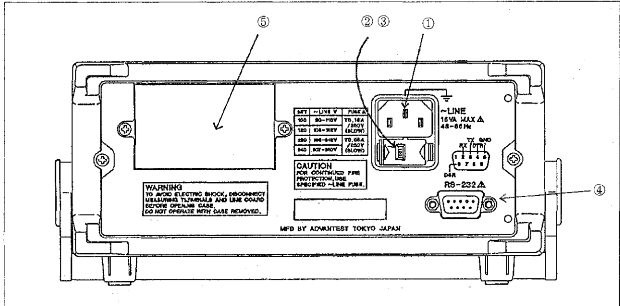
図 3 - 5 背面パネルの説明
